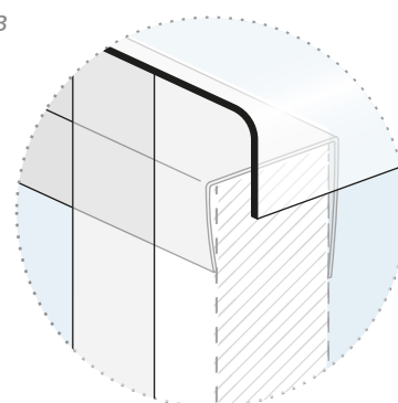
OPZIONE B OPTION B Lato lungo interno Internal long side
