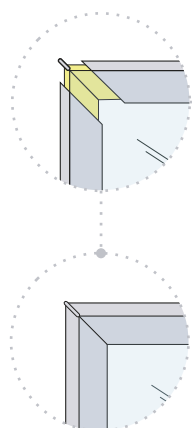
FBS 9444 Assemblaggio con flangia Assembly with flange
