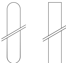
Raggio a 3 mm Taglio a 90° 3 mm radius 90° cut
