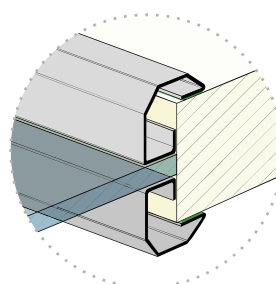
FERMAVETRI GLASS FIX
